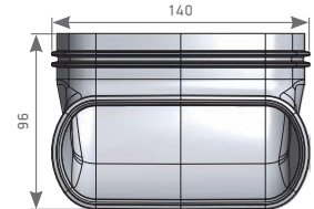
Вертикальный переходник 90°
