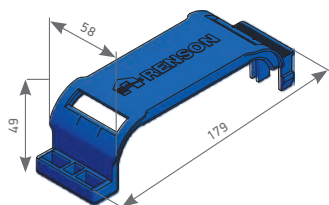
Защелка
